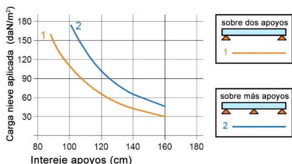
CARGAS GRECA 28/112 esp. 6 mm APLICACIÓN PLANA
