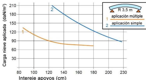
CARGAS GRECA 28/112 esp. 6 mm APLICACIÓN CURVA R3500 mm
