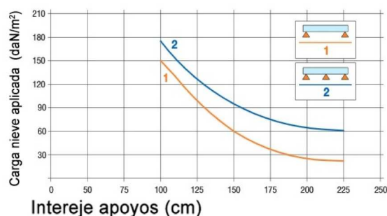
APLICACIÓN PLANA SOBRE DOS O MÁS APOYOS
