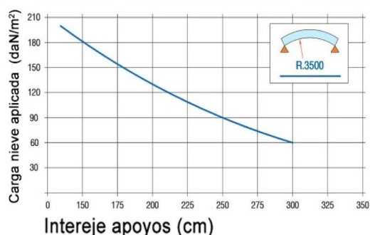
APLICACIÓN CURVA R3500
