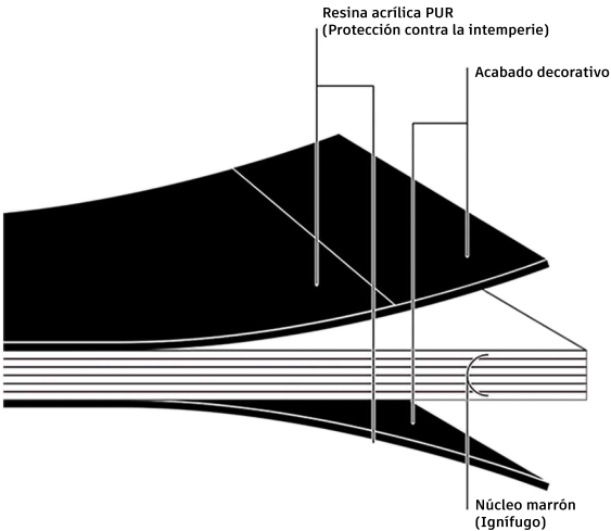
Estructura panel Max Compact Exterior
